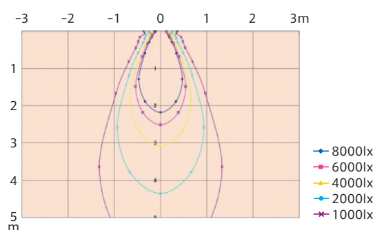
鉛垂照度分布 (1台当たり) 水平方向
